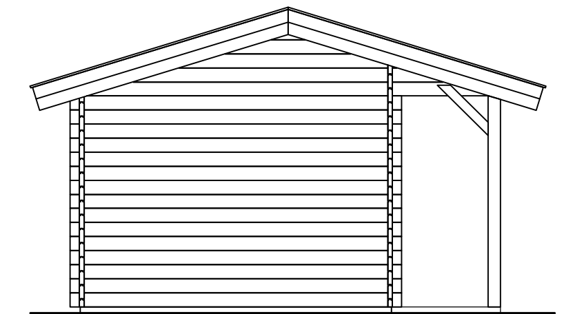
zij aanzicht (l) side view (l)
