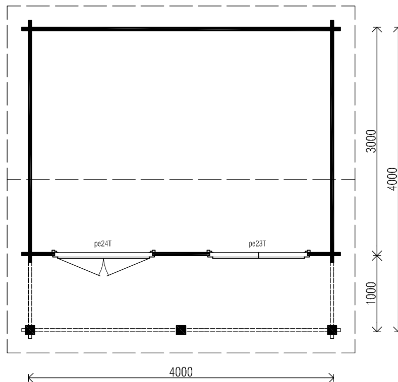
plattegrond / plan
